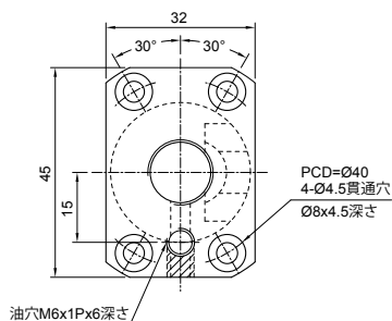
D 矢視
