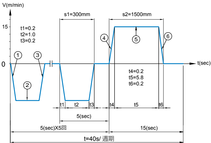
図37. 垂直運搬装置 v-tダイアグラム
